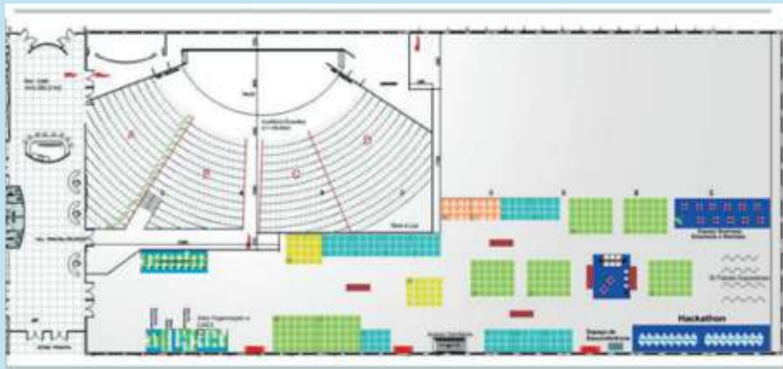
Planta baixa do Centro de Eventos FAURGS
